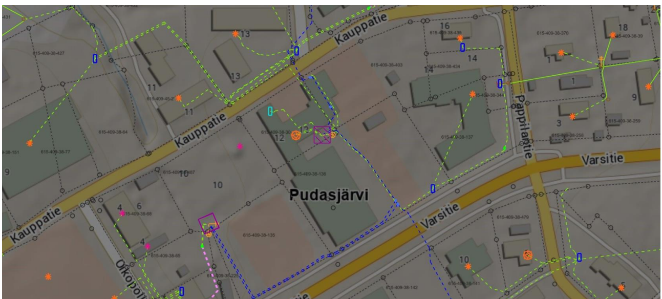
Alueen sähköverkkoa kuvaava kartta. 20 kV johdot ovat sinisellä ja 0,4 kV johdot vihreällä ja vaaleanpunaisella värillä. Ilmajohdot on esitetty yhtenäisellä viivalla ja maakaapelit katkoviivalla. Puistomuuntamot ovat violetteja neliöitä.
